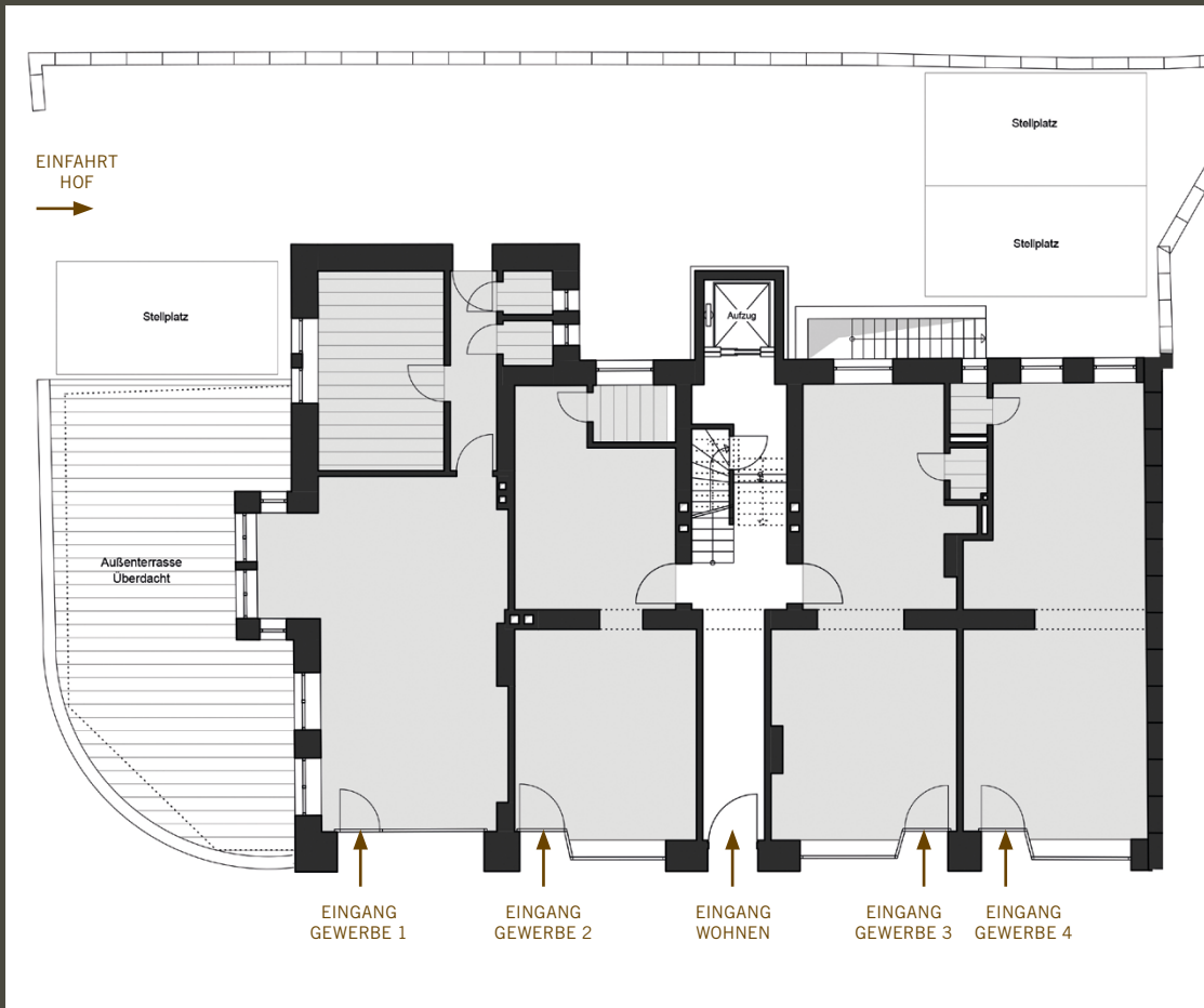
LAGEPLAN ERDGESCHOSS MIT HOF
